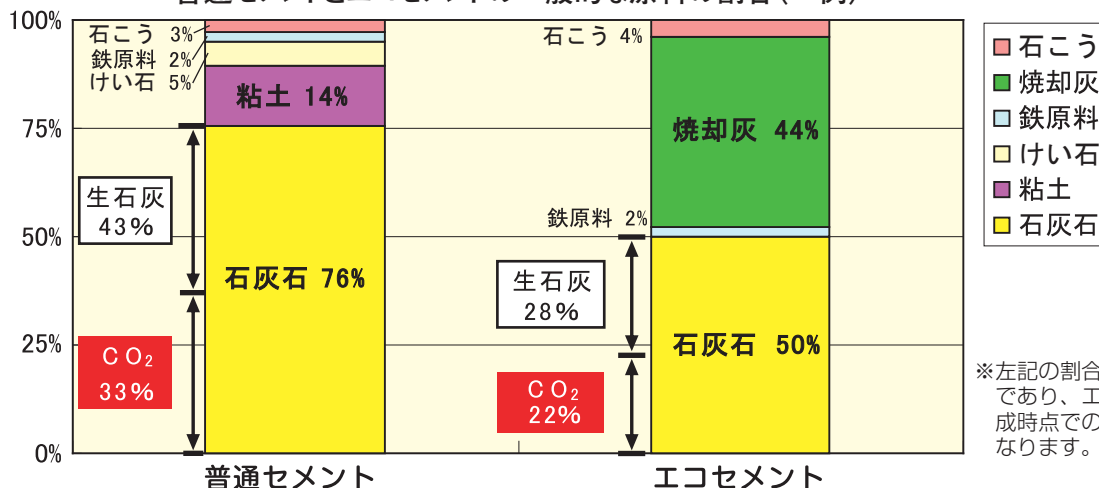
普通セメントとエコセメントの一般的な原料の割合（一例）
