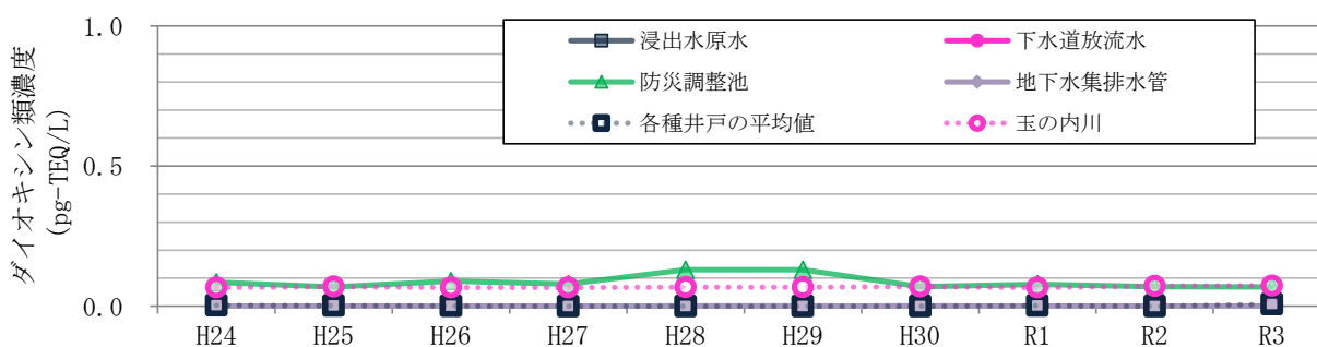
図-4 ニツ塚処分場・水中のダイオキシン類濃度の経年変化 (過去10年) (調査地点種別ごとの平均値の推移)
