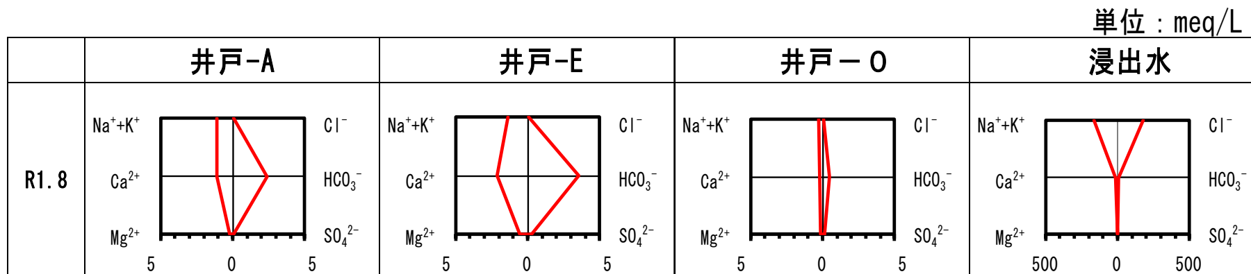
図-2 モニタリング井戸のイオンバランス
