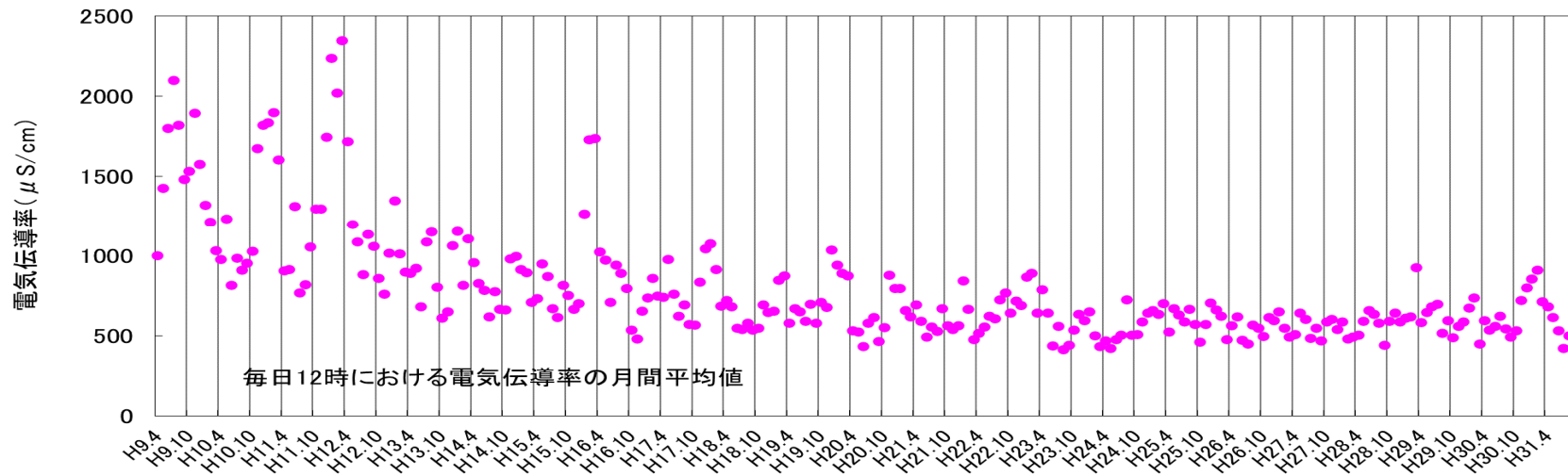
図-1 地下水No. 2の電気伝導率の変化
