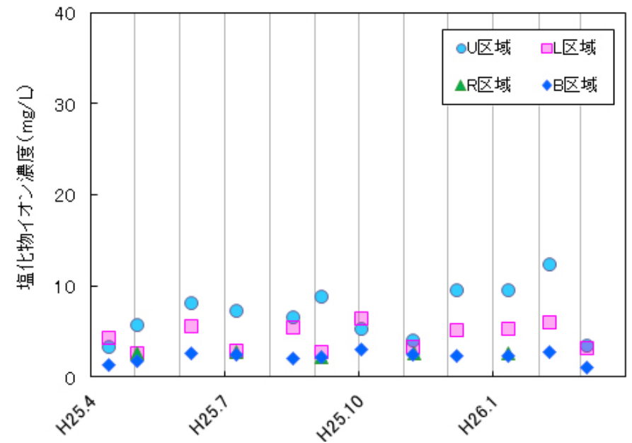
図-5 測定頻度見直し後の下流部観測孔各区域における塩化物イオン濃度（平均値）
