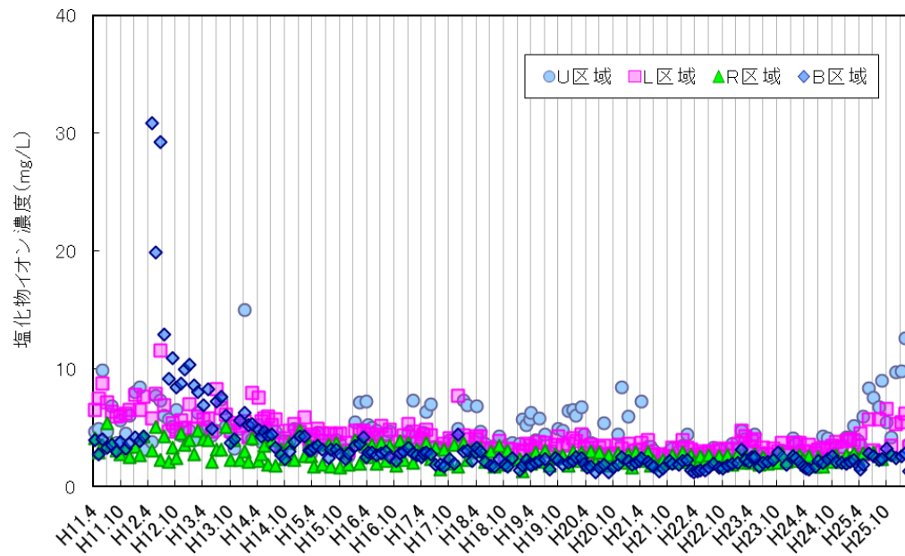
図-4 下流部観測孔各区域における塩化物イオン濃度（平均値）
