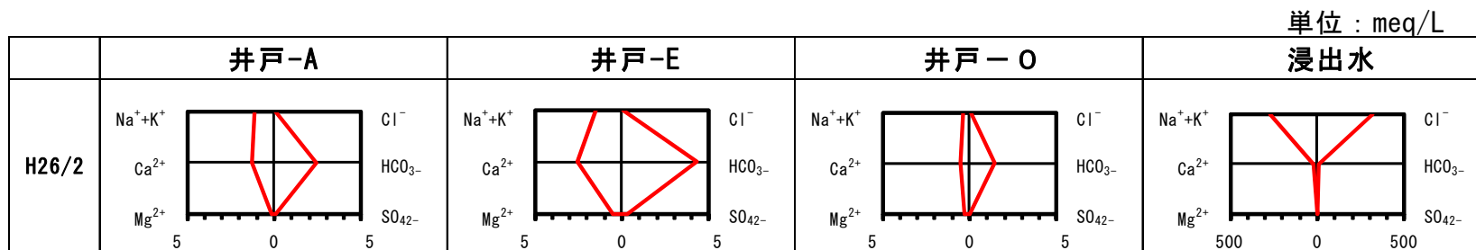
図-2 場内モニタリング井戸のイオンバランス
