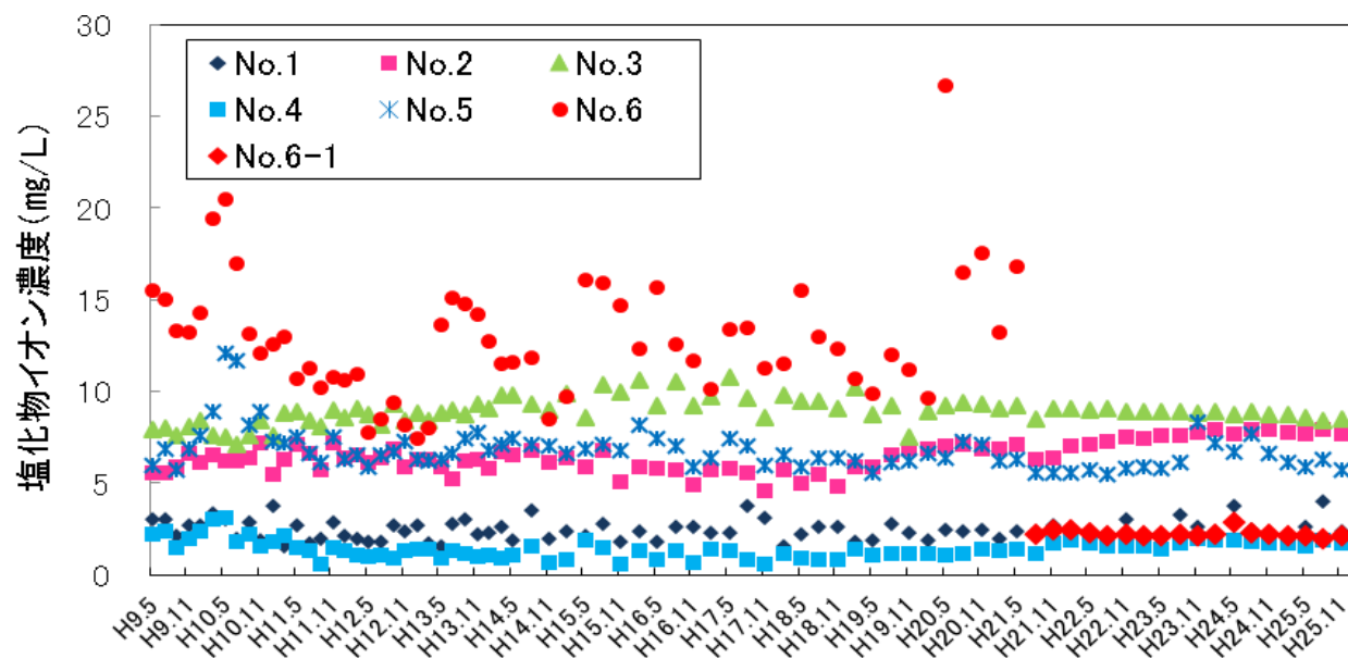
図-2 場内モニタリング井戸の塩化物イオン濃度の推移
