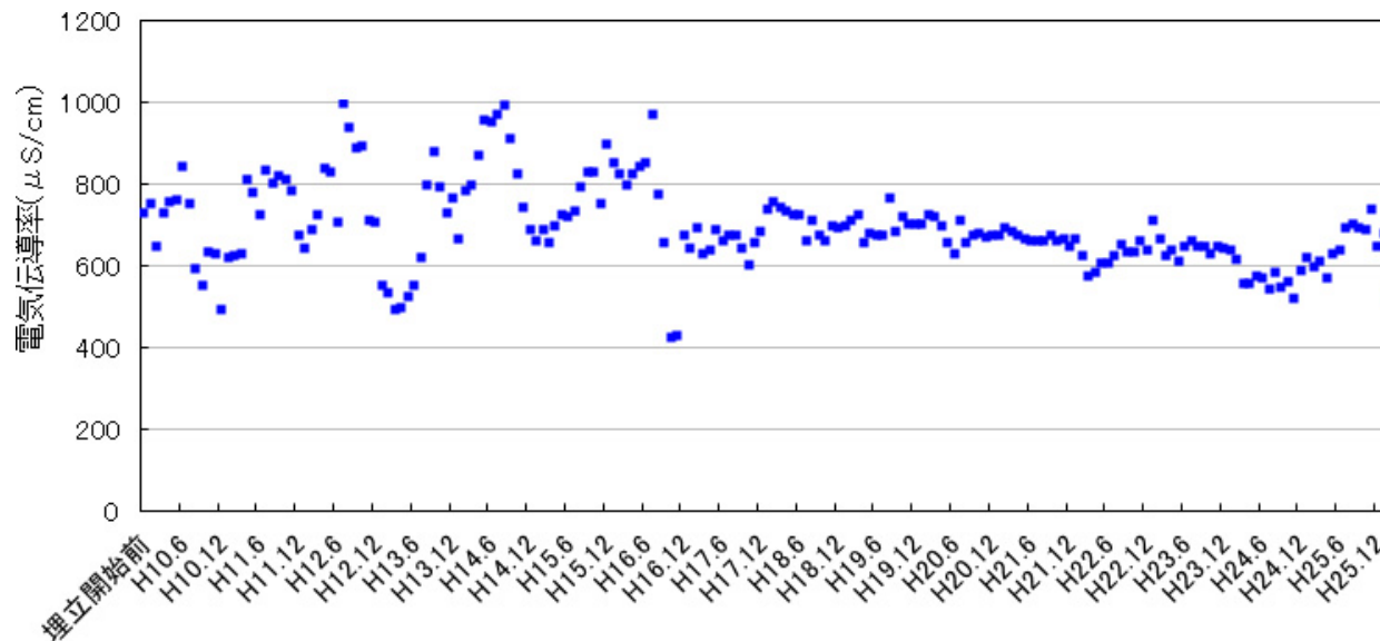
図-1 地下水集排水管水の電気伝導率の推移
