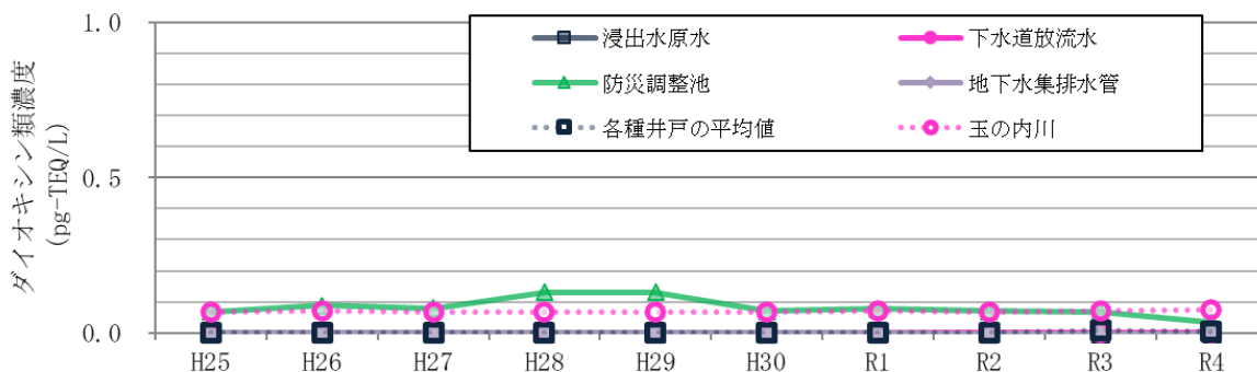
図-4 ニツ塚処分場・水中のダイオキシン類濃度の経年変化 (過去10年) (調査地点種別ごとの平均値の推移)
